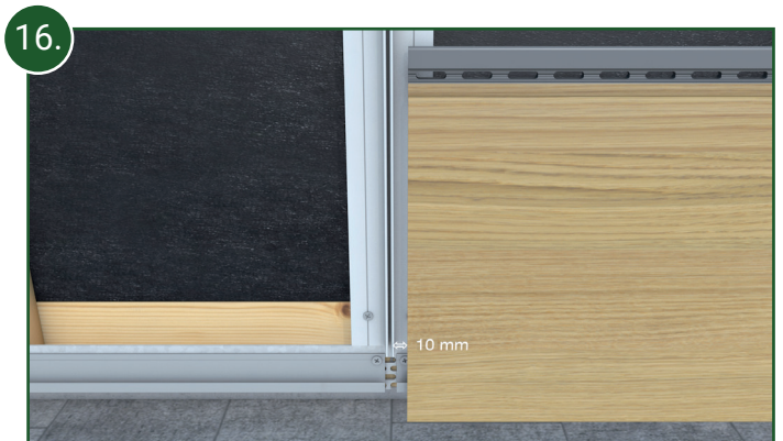
16. Der Dehnabstand zwischen den Enden der Fassadenprofile und den Enden der 2-teiligen Verbindungs-, Abschluss- und Eckprofile sowie des variablen Eckprofils muss jeweils 10 mm pro Seite betragen (siehe Skizze)!
